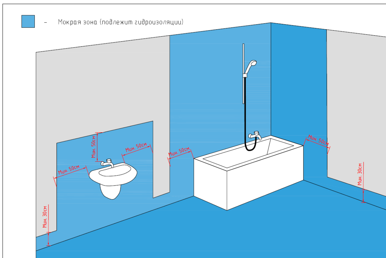
28.2 Мокрые зоны внутри влажных помещений, подлежащие гидроизоляции.
