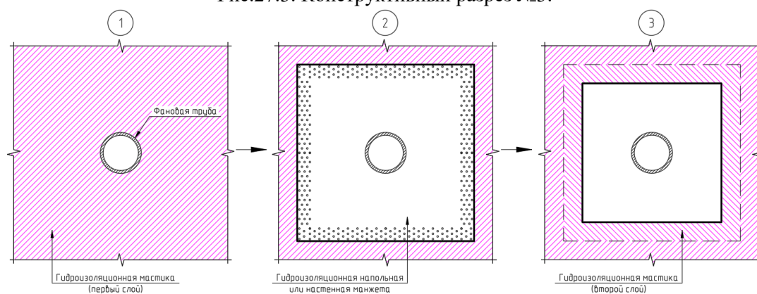
Рис.27.4. Последовательность нанесения гидроизоляционной манжеты.
