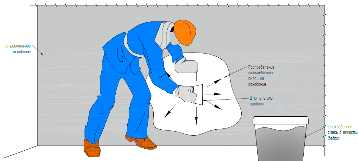
Рис. 30. Организация работ по нанесению шпаклевочной смеси
